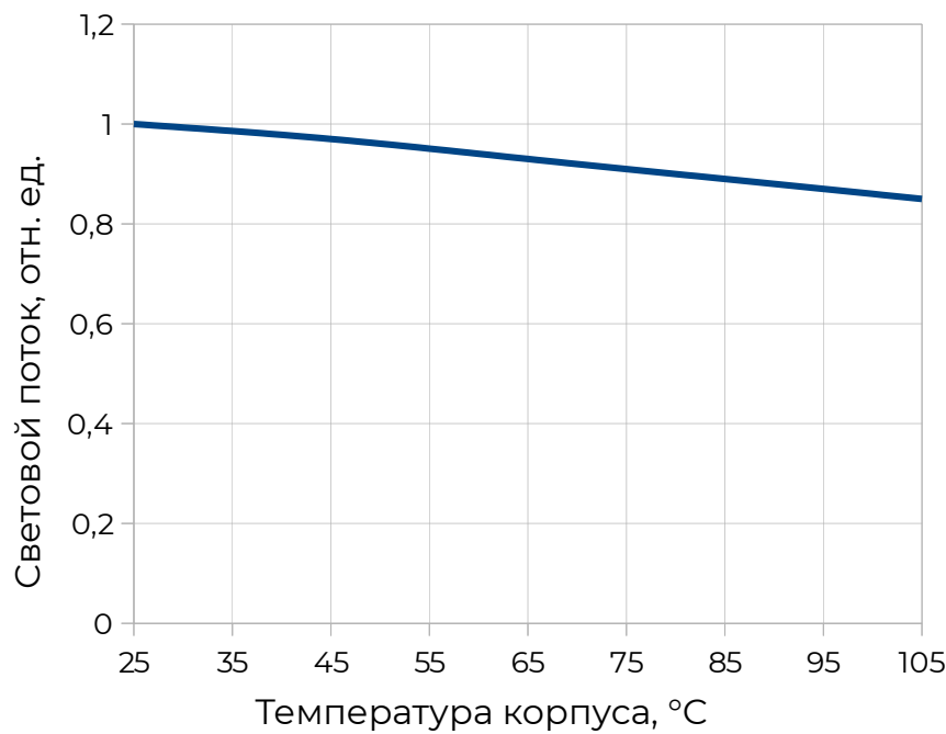
Зависимость светового потока от температуры перехода (IF = 150мА, Tj = 25 °С)
