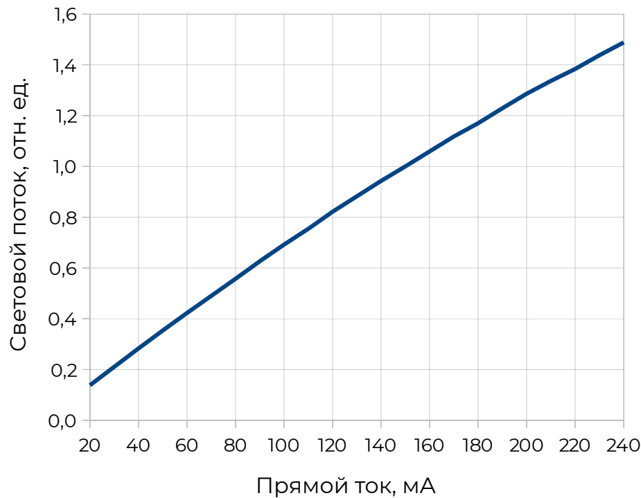
Зависимость светового потока от прямого тока (Tj = 25 °С)
