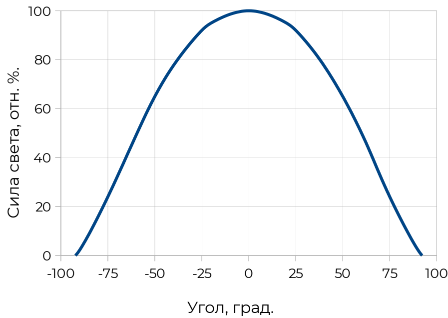
Кривая силы света (IF = 150мА, Tj = 25 °С)
